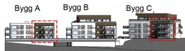
Fasade øst
